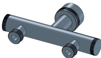
Adattatore tramoggia due uscite Hopper adaptor with two exits 12.A1
