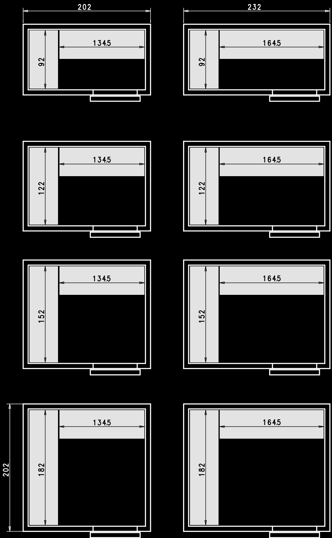
COMPOSIZIONE CELLE CON SCAFFALATURE LAYOUT OF COLD ROOMS WITH SHELVES
